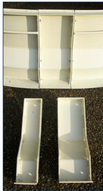
Coffrages centraux de 100,150 et 200
